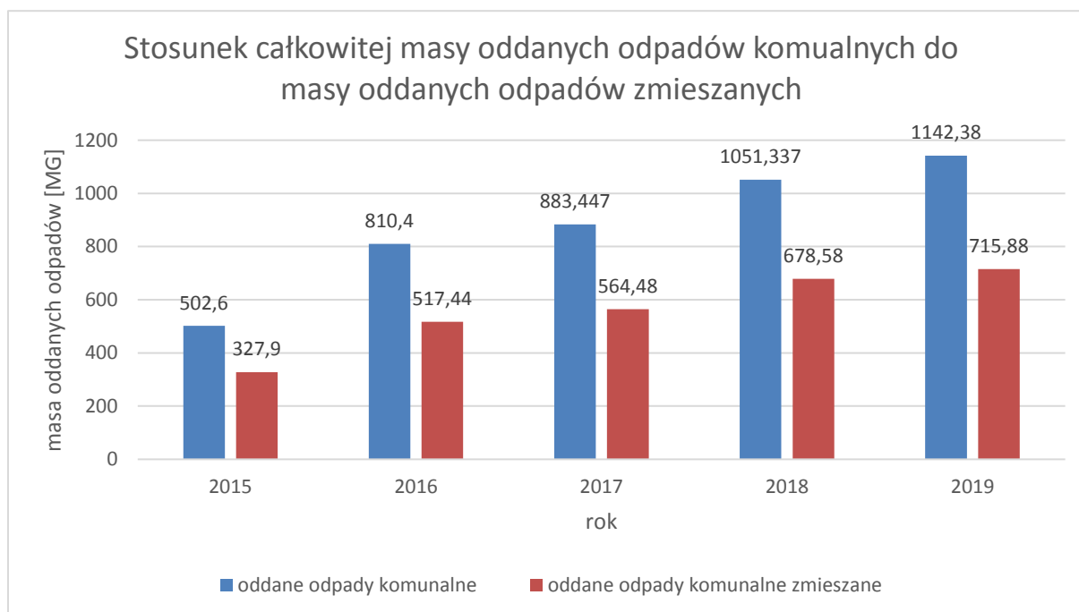
Wykres 3. Ilość oddawanych odpadów z podziałem na poszczególne frakcje
