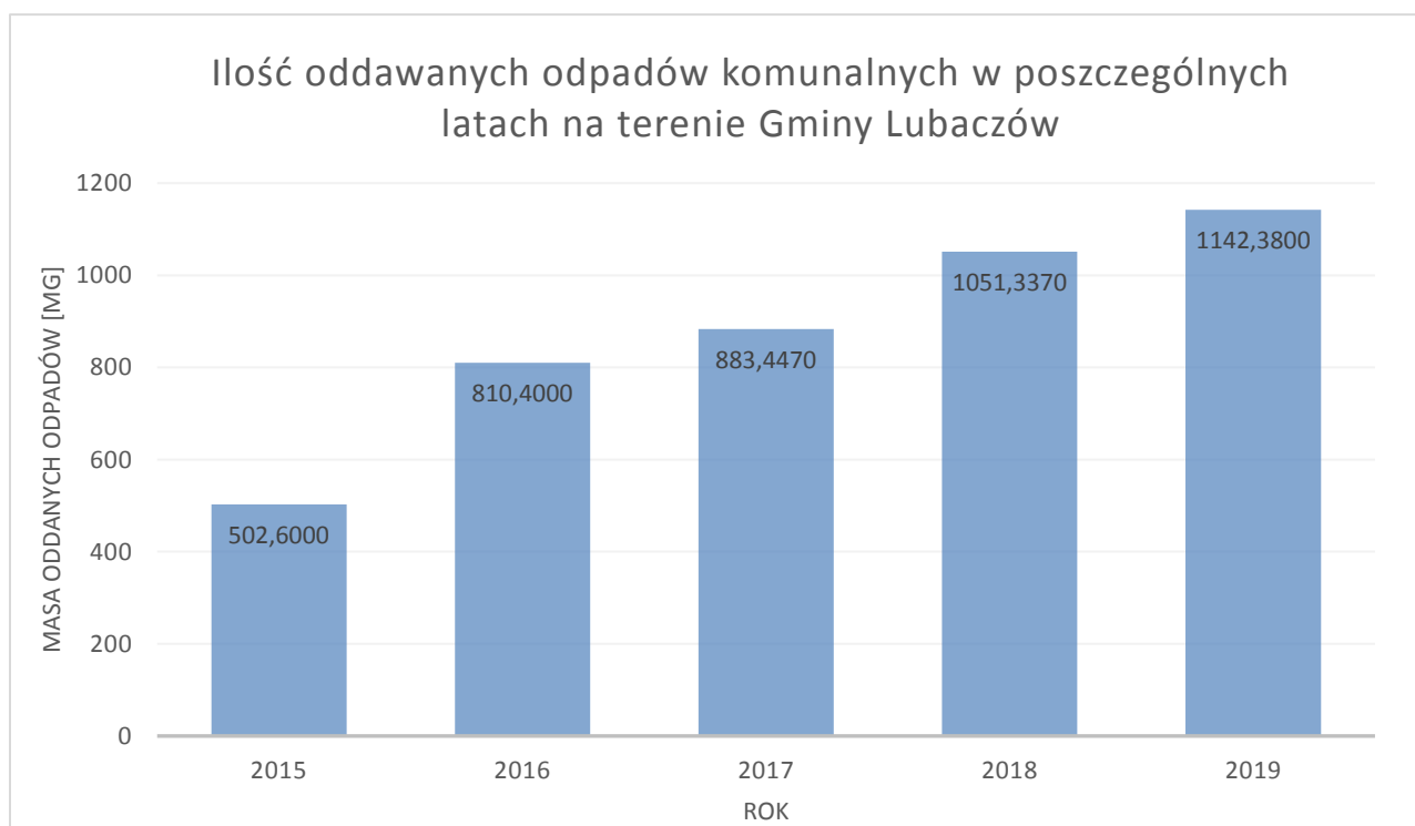
Wykres 1. Ilość oddawanych odpadów komunalnych w latach 2015-2019r. na terenie Gminy Lubaczów
